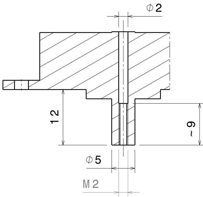
A-A section
