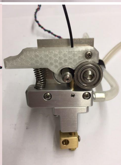
Ganzmetall – Direktextruder Wassergekühlt, 1,75mm Didischu , 29.012019 ( vw-styler , Rep Rap Forums )
