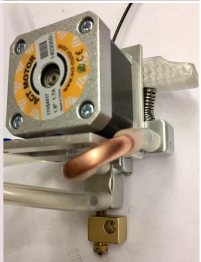
Ganzmetall – Direktextruder Wassergekühlt, 1,75mm Didischu , 29.012019 ( vw-styler , Rep Rap Forums )
