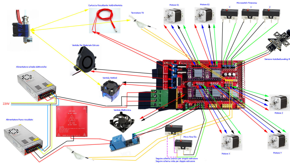
Figura 1 - Schema generale dei collegamenti
